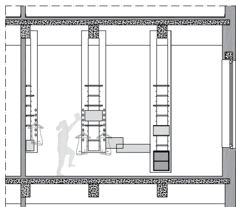
COUPES SUR LE MAGASIN DIDACTIQUE
